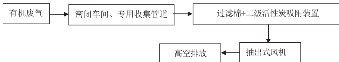
图2-3 有机废气处理工艺流程图
